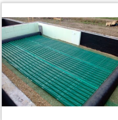
Gruntowy wymiennik ciepła GEOSTRONG – w fundamentach. GWC bezprzeponowy modułowy. Przepływ powietrza turbulenty, wymiana cieplna ze wszystkich stron GWC. Wytrzymałość na nacisk z góry: 460 t/m 2 . Zastosowanie: w wentylacji mechanicznej we współpracy z rekuperatorem w domach jednorodzinnych, wielorodzinnych i przemyśle. Możliwość wykonania GWC o każdej wielkości przepływu powietrza. Możliwość samodzielnego montażu.
