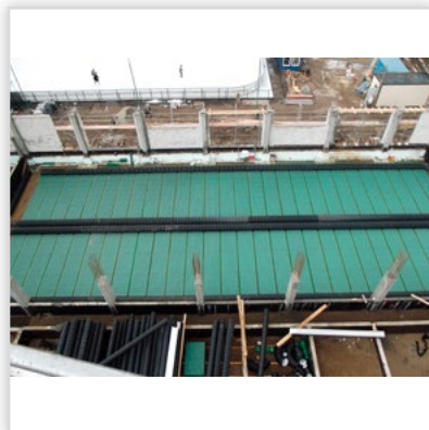
Gruntowy wymiennik ciepła GEOSTRONG – w fundamentach rozstrzelony dla hali sportowej
